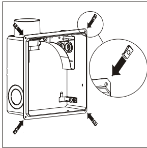
A gyorsrögzítőket rátolni a ventilátorház sarkaira
